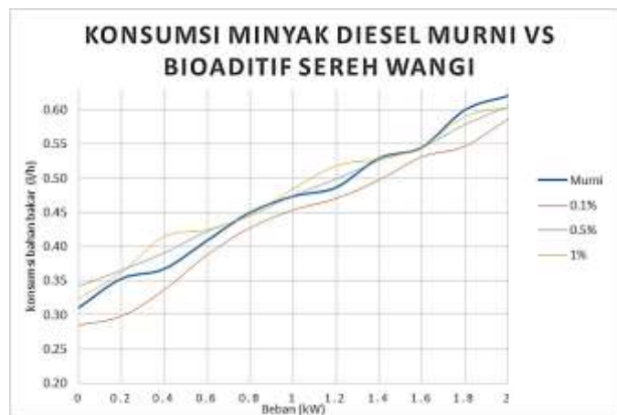
Gambar 5. Grafik perbandingan konsumsi bahan bakar dari pemakaian minyak diesel murni berbanding bioaditif serreh wangi
