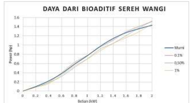
Gambar 1. Grafik perbandingan daya dari pemakaian minyak diesel murni berbanding bioaditif serah wangi.
