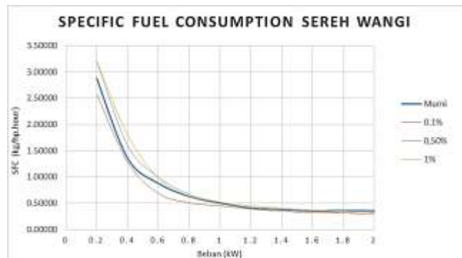
Gambar 4. Grafik perbandingan SFC dari pemakaian minyak diesel murni berbanding bioaditif serreh wangi
