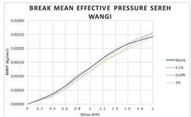
Gambar 3. Grafik perbandingan BMEP dari pemakaian minyak diesel murni berbanding bioaditif serah wangi
