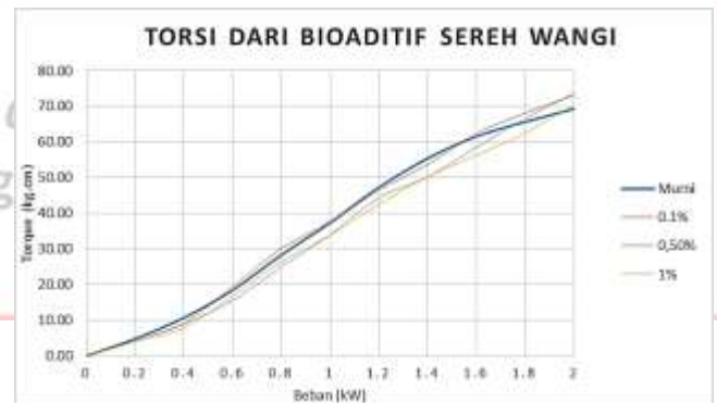
Gambar 2. Grafik perbandingan torsi dari pemakaian minyak diesel murni berbanding bioaditif serah wangi
